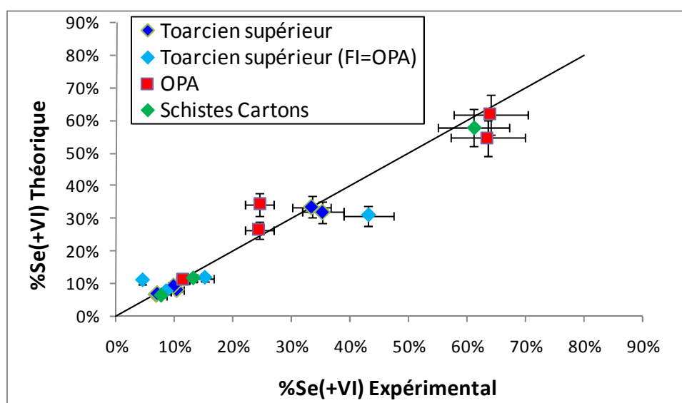
Figure 47 : Comparaison entre la spéciation du Se déterminée expérimentalement et la spéciation du Se théorique
