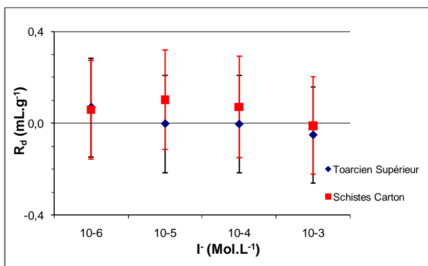
Figure 3 : Isothermes de sorption des iodures dans le Toarcien supérieur et les Schistes Cartons en conditions oxygènes suite à une semaine d'équilibration.
