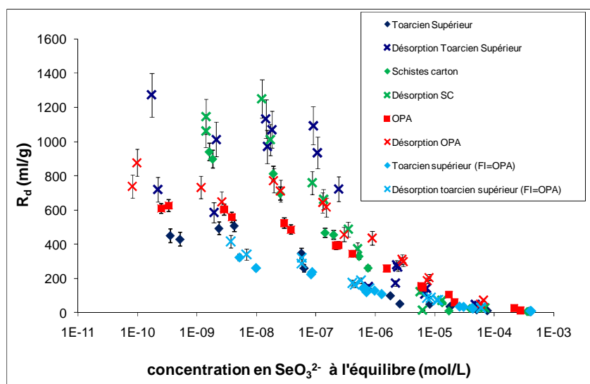
Figure 92 : Comparaison des isothermes de sorption aux isothermes de désorption dans les argilites du Toarcien supérieur, les argilites du Toarcien supérieur avec FI=OPA, l'OPA et dans les Schistes Cartons
