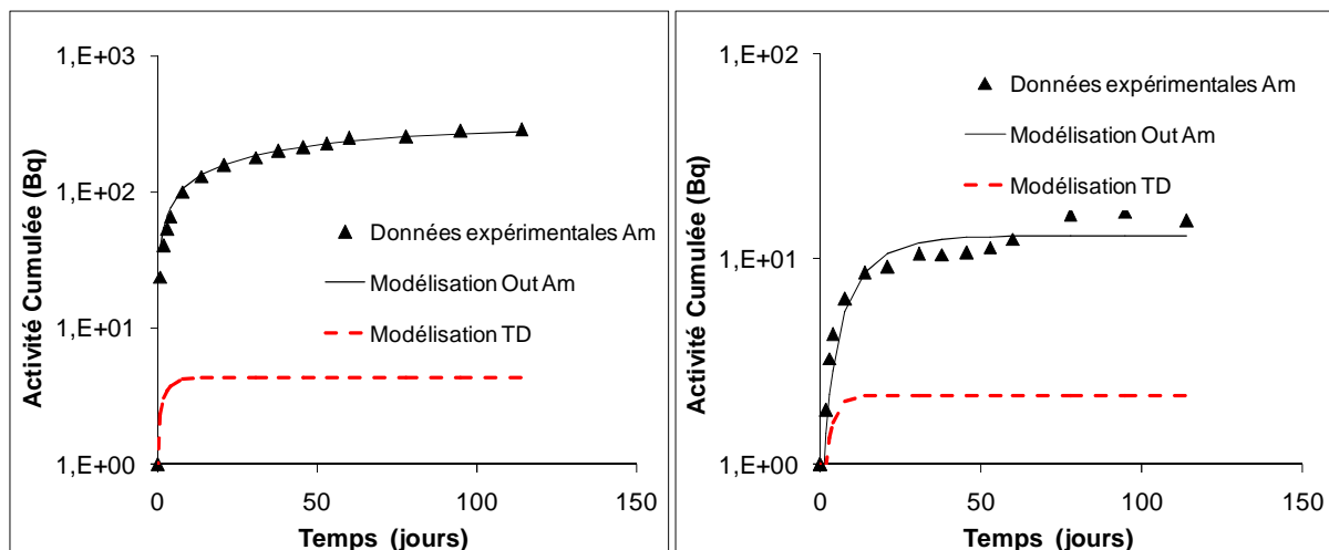
Figure 43 : Comparaison des résultats d'out-diffusion avec des modélisations calibrées sur les résultats de through-diffusion obtenus sur l'échantillon PH4-37-1 (BAG, [I]=10^{-6} \text{ mol}\cdot\text{L}^{-1} )
