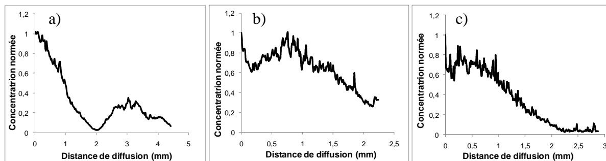
Figure 78 : Profils de diffusion du Se acquis sur différentes sections dans l'échantillon PH4-37-10
