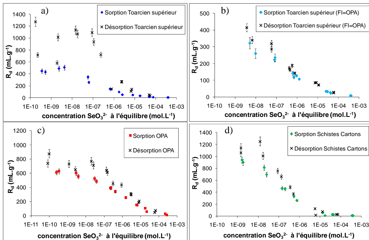
Figure 52 : Isothermes de désorption des sélénites dans (a) les argillites du Toarcien supérieur, (b) les argillites du Toarcien supérieur avec FI=OPA, (c) dans l'OPA, (d) dans les Schistes Cartons
