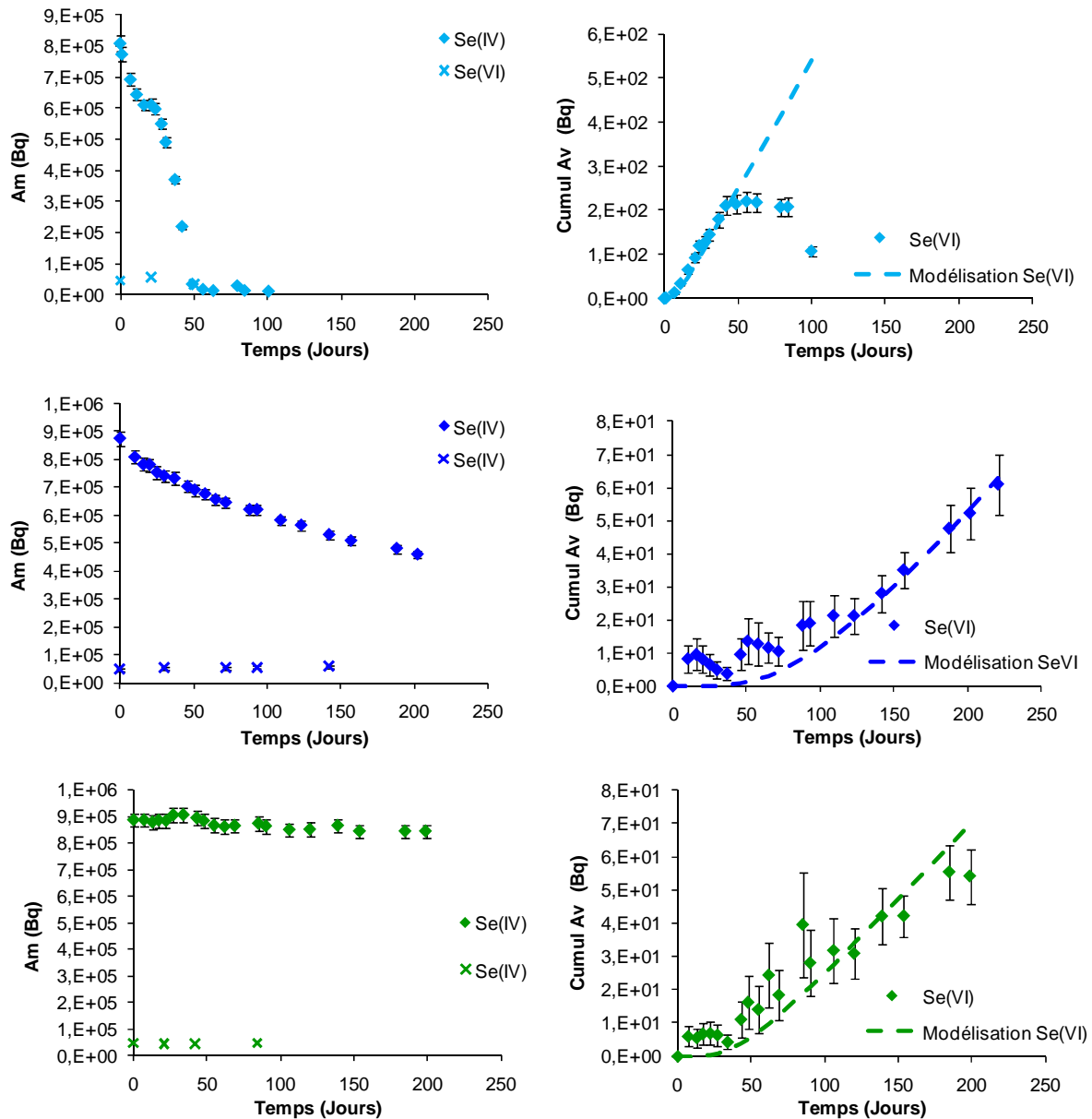
Figure 66 : Données expérimentales en solution du ^{75}\text{Se} obtenues dans les échantillons PH4-37-5(a), PH4-37-6(b) et PH4-37-7(c): les graphiques de gauche représentent les activités amont et ceux de droite les activités cumulées aval
