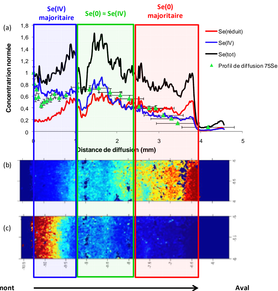
Figure 104 : Profil de diffusion du sélénium en inactif ainsi que profil de diffusion du Se(IV) obtenu en actif dans l'échantillon BDR0-2 (a), cartes redox des concentrations relatives en Se(IV) (b) et en Se réduit (c)
