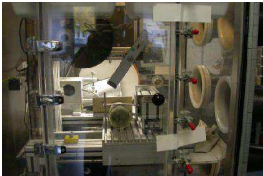
Figure 18 : Photo de la carotte 3715 (forage PH4) lors de sa découpe à la scie à fil en boîte à gants anoxique.
