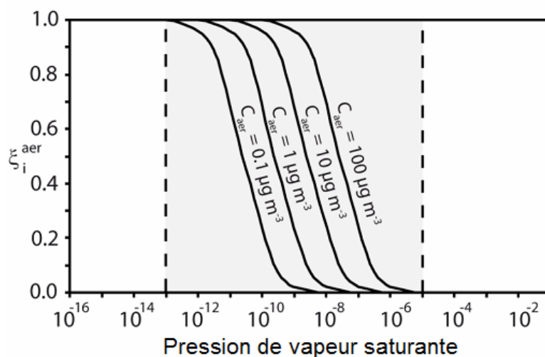
Figure V- 35 : Fraction \xi_{aer,i} d'une espèce i semi-volatile en phase condensée à l'équilibre thermodynamique avec la phase gazeuse, en fonction de sa pression de vapeur saturante pour des conditions atmosphériques typiques. D'après Valorso et al., (2011).
