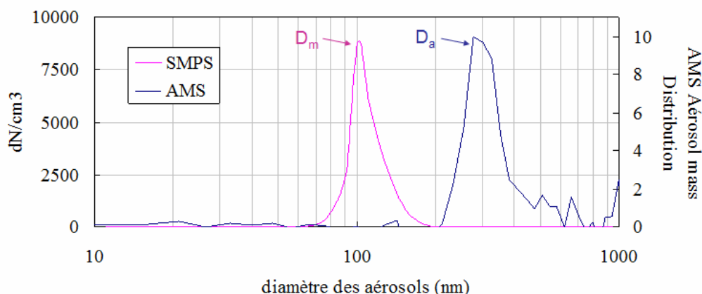
Figure V- 32 : Distributions granulométriques des aérosols mesurées par SMPS et AMS à 166 min (expérience 9)
