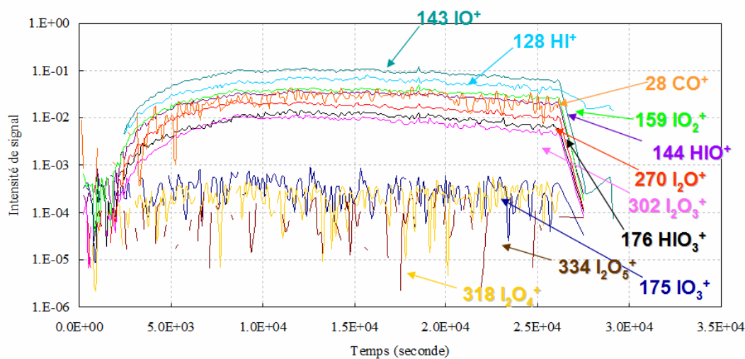
Figure V- 27 : Evolution des fragments IO^+ , CO^+ , HI^+ , IO_2^+ , HIO^+ , I_2O^+ , HIO_3^+ , I_2O_3^+ , I_2O_4^+ , I_2O_5^+ et IO_3^+ en fonction du temps lors de l'expérience 9
