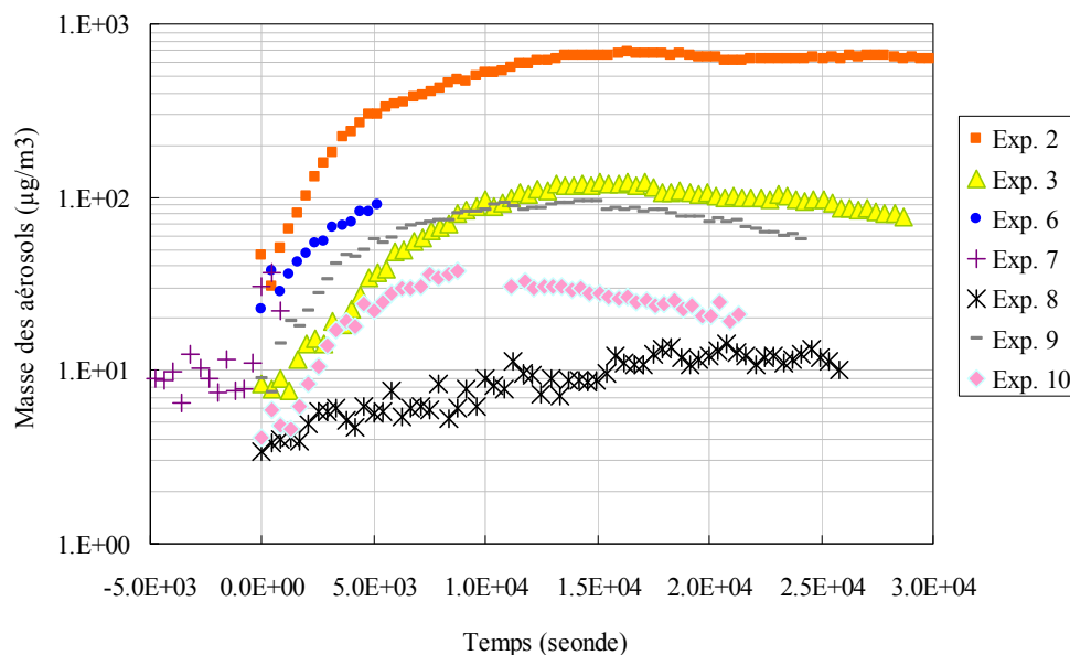
Figure V- 22 : Comparaison de la masse totale d'aérosols pour différentes concentrations de CH 3 I (15ppb pour exp 2, 3 et 7 et 45 ppbV pour exp 6, 9 et 10). [exp 8 CH 3 I 15+15 ppbV]
