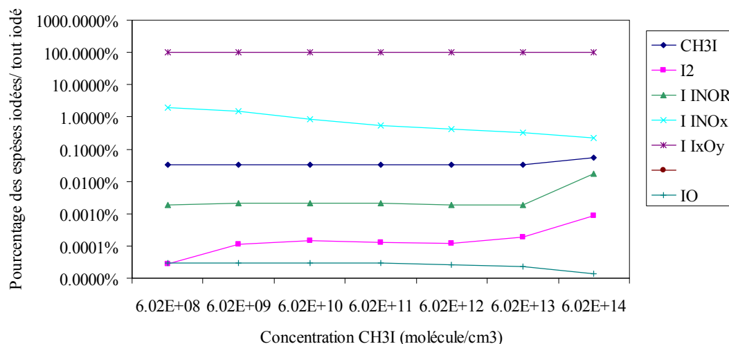
Figure IV- 8 : Pourcentages moyens des espèces iodées sur le temps total étudié en fonction de la concentration initiale CH 3 I à 90°C, humidité relative à 80% et débit de dose de 36kGy/h
