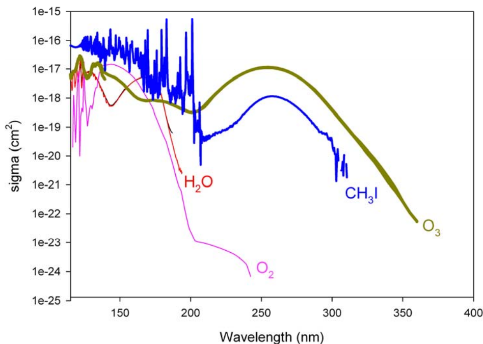
Figure V- 4: Sections efficaces des espèces du milieu réactionnel (Ackerman 1971) (Eden, Limão-Vieira et al. 2006)
