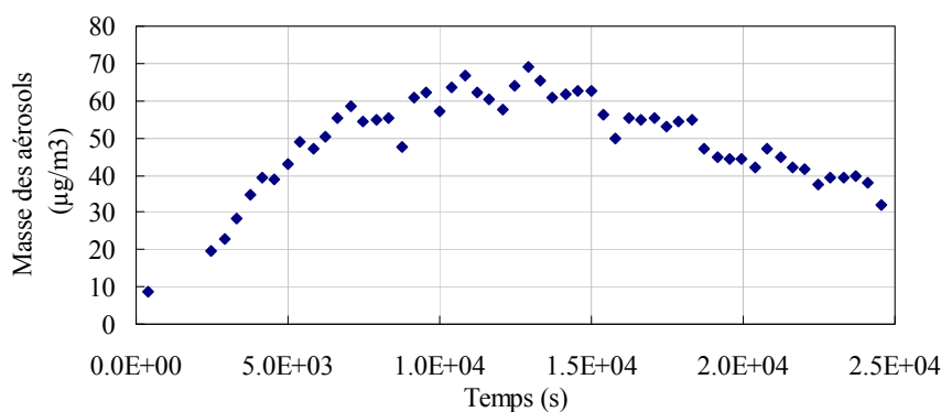
Figure V- 34 : Concentration massique réelle des aérosols en fonction de temps pour l'expérience 9, calculée à partir de l'équation précédente et de la densité expérimentale (Figure V- 33)
