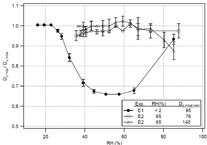
Figure II- 16: Facteur hygroscopique des aérosols d'oxydes d'iode (Jimenez 2003)
