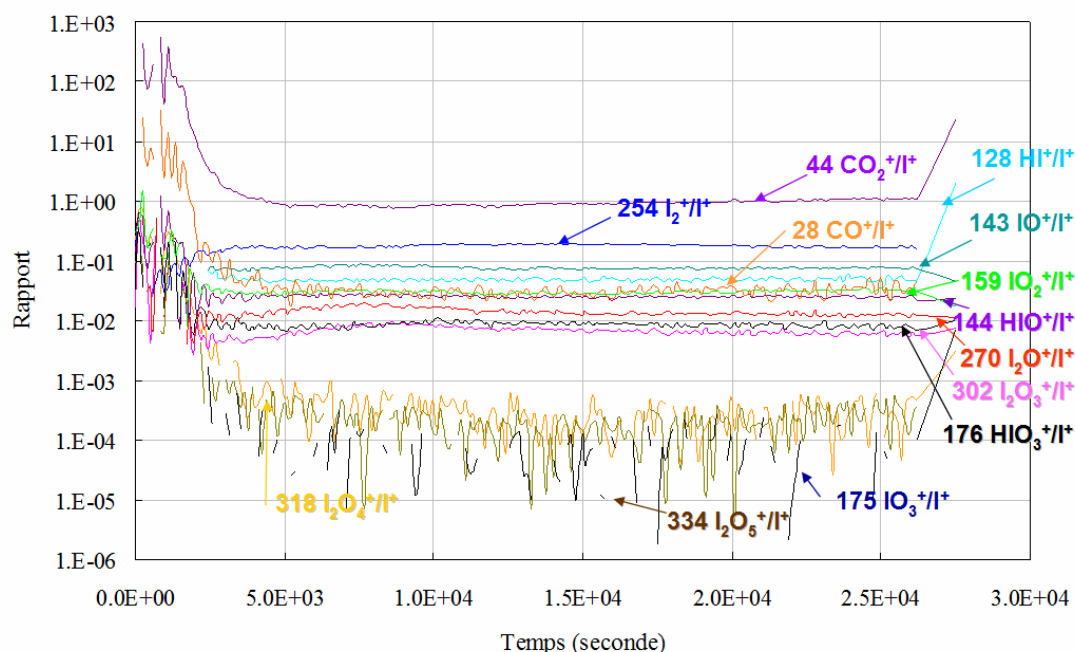
Figure V- 28 : Ratio des signaux des fragments des aérosols d'oxydes d'iode par rapport au signal de I^+ lors de l'expérience 9
