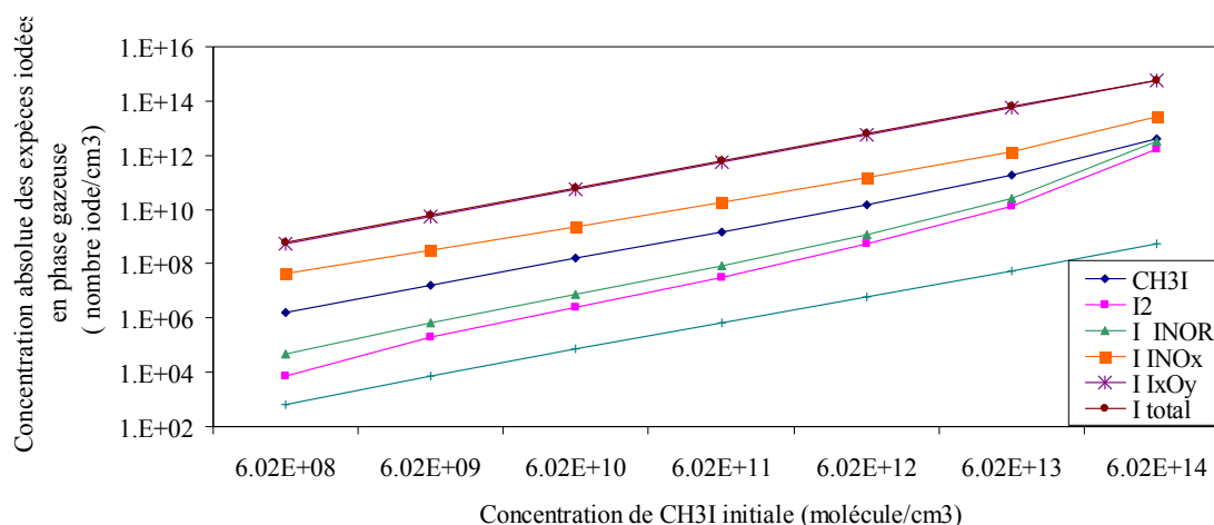
Figure IV- 5 : Concentrations moyennes des espèces iodées sur le temps total étudié en fonction de la concentration initiale de CH 3 I, à 90°C, humidité relative à 80% et débit de dose de 3.6kGy/h
