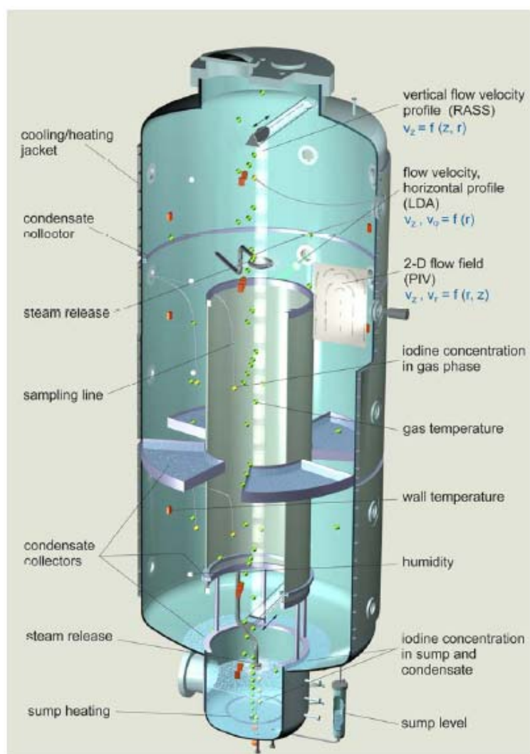
Figure II-7 : schéma et instrumentation de l'installation ThAI
