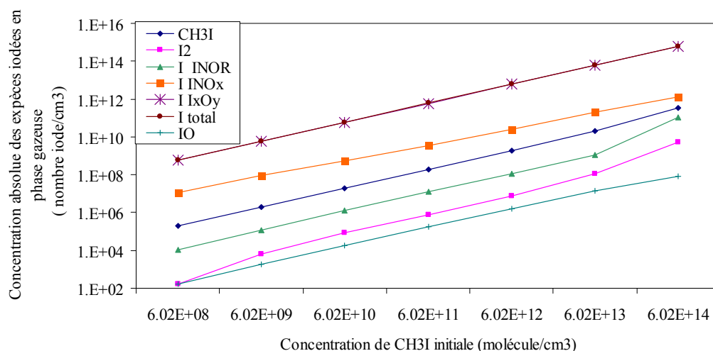
Figure IV- 7 : Concentrations moyennes des espèces iodées sur le temps total étudié en fonction de la concentration initiale CH3I, à 90°C, humidité relative à 80% et débit de dose de 36kGy/h
