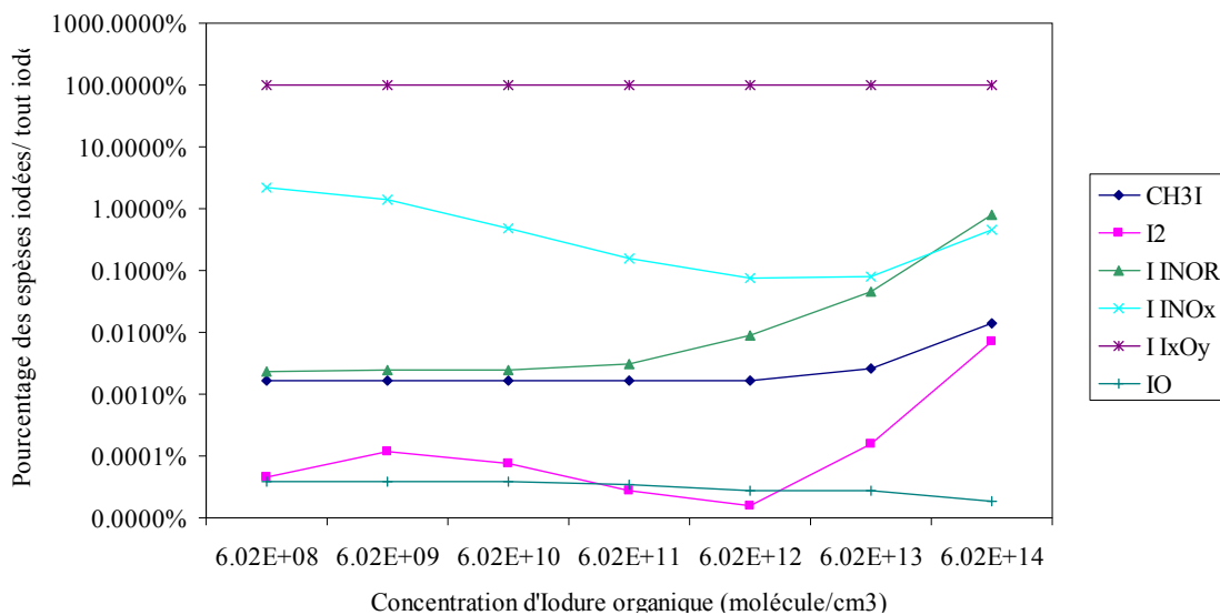
Figure IV- 10 : Pourcentages moyens sur le temps total des espèces iodées en fonction de la concentration initiale des iodures organiques à plus longue chaîne, à 90°C, humidité relative à 80% et débit de dose de 36kGy/h
