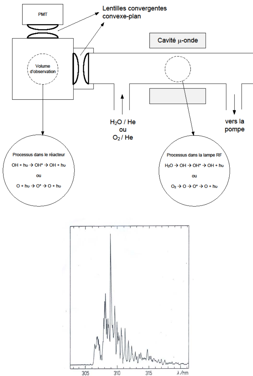
Figure III- 4 : Schéma de la lampe (gauche) et spectre de la lampe RF à 308nm, radical OH ( A^2\Sigma^+ \rightarrow X^2\Pi ).
