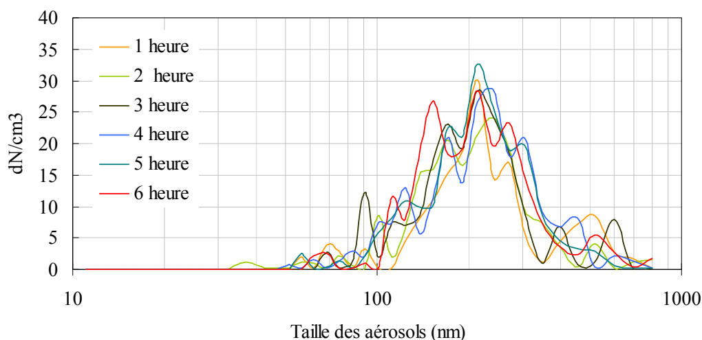
Figure V- 8 : Distribution granulométrique des aérosols en nombre (mesurée par le SMPS) lors de l'expérience 1, durant 6h. \text{CH}_3\text{I} 15ppb, HR 60%, \text{O}_3 1ppm, à 30°C SANS photolyse (dans le noir)
