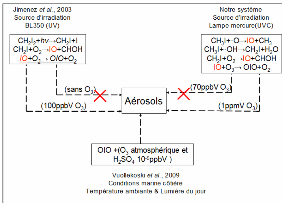
Figure V- 23 : Conditions nécessaires à la nucléation des aérosols d'oxydes d'iode des différentes expériences
