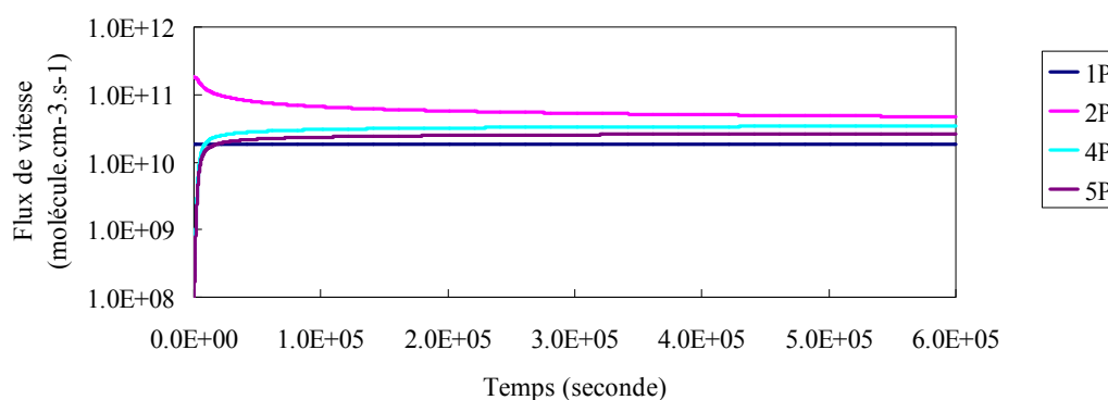
Figure IV- 4 : Flux de vitesse des réactions productrices de ·O, les plus importantes dans les conditions standards.
