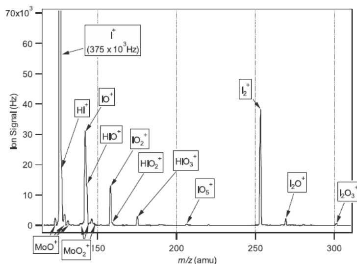
Figure II-14 : Composition des aérosols avec 50ppb de \text{CH}_2\text{I}_2 , 500ppb de \text{O}_3 et une humidité relative inférieure à 2% à température ambiante (D.O'Dowd 2002) (Jimenez 2003)
