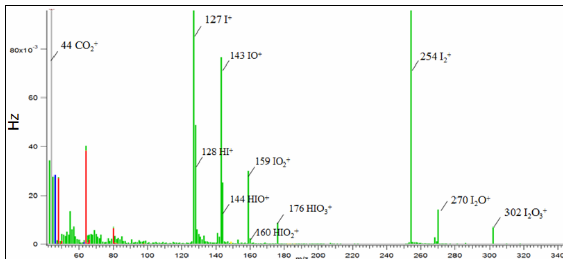
Figure V-24: Spectre moyen de masse des aérosols (sur la durée totale) mesuré par HR-ToF-AMS lors de l'expérience 9
