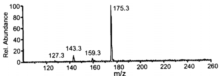
Figure II-13 : Masse des fragments des aérosols d'oxydes d'iode observée par (Hoffmann 2001)
