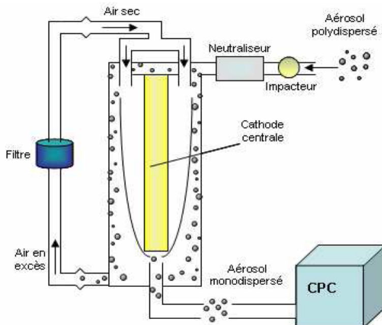
Figure V- 5 : Schéma de principe de la colonne DMA
