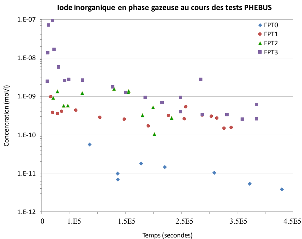
Figure II-2 : concentration d'iode inorganique dans l'enceinte PHEBUS pour FPT0, FPT1, FPT2 et FPT3 ( \text{mol.L}^{-1} )
