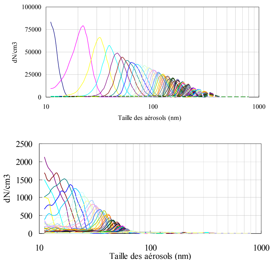
Figure V- 17: Comparaison du nombre et de la taille des particules entre les expériences 2 (en haut : HR 60%) et 4 (en bas : HR 15%).
