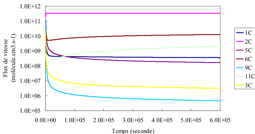
Figure IV- 1 : Flux de vitesse des réactions consommatrices de ·OH les plus importantes dans les conditions standards
