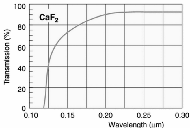
Figure III- 8 : Spectre de transmission de la fenêtre CaF 2
