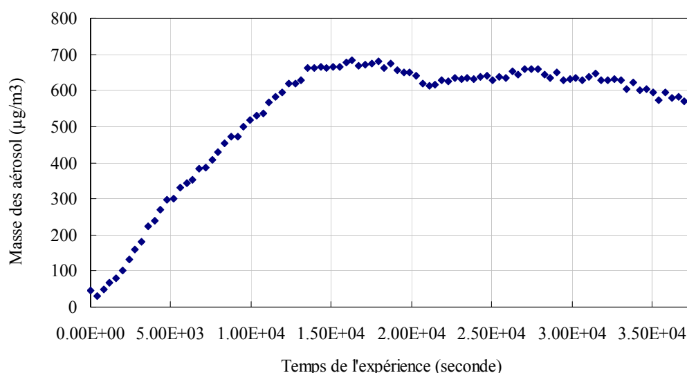
Figure V- 12 : Evolution de masse totale des aérosols pour l'expérience 2, \text{CH}_3\text{I} 15ppb, HR 60%, \text{O}_3 2ppm, à 30^\circ\text{C} avec photolyse (sans correction de la dilution, due aux flux d'air entrants et sortants, et en supposant une densité de 4\ \text{g/cm}^3 )
