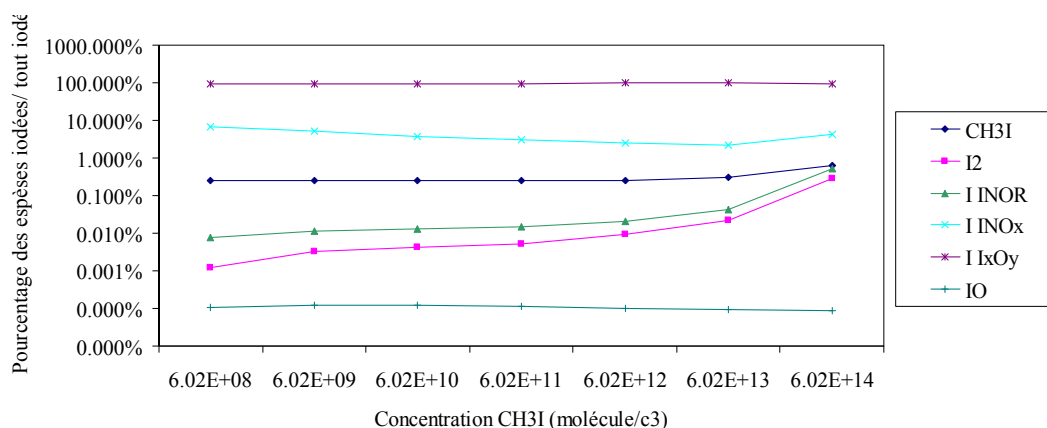
Figure IV- 6 : Pourcentages moyens (par rapport à I total) des espèces iodées sur le temps total étudié en fonction de la concentration initiale CH3I à 90°C, humidité relative à 80% et débit de dose de 3.6kGy/h
