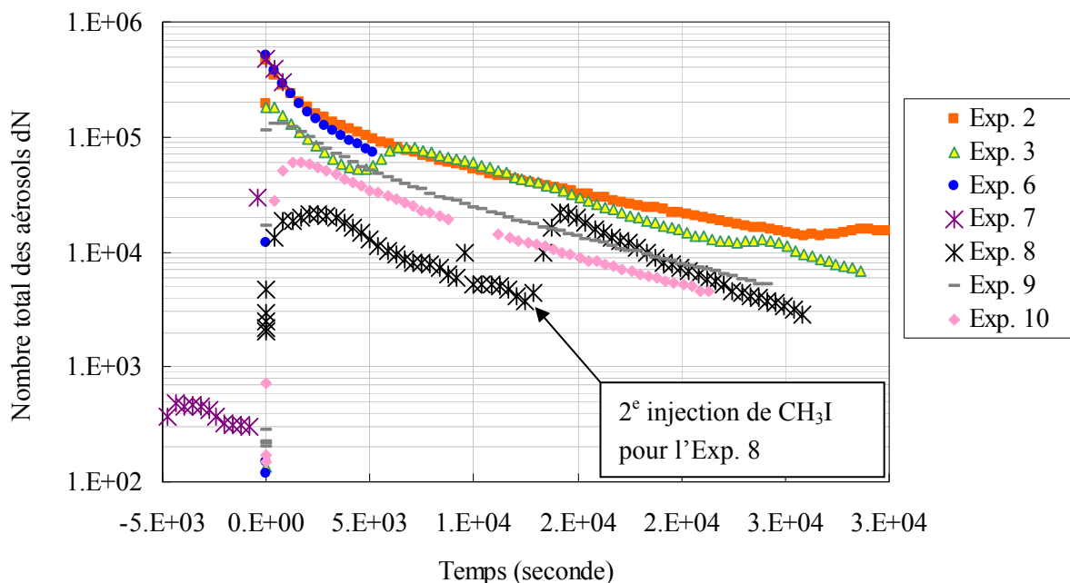
Figure V- 21 : Comparaison du nombre totale d'aérosols pour différentes concentrations de \text{CH}_3\text{I} (15ppbV, pour exp 2, 3 et 7, et 45 ppb pour exp 6, 9 et 10). [exp 8 \text{CH}_3\text{I} 15+15 ppbV]
