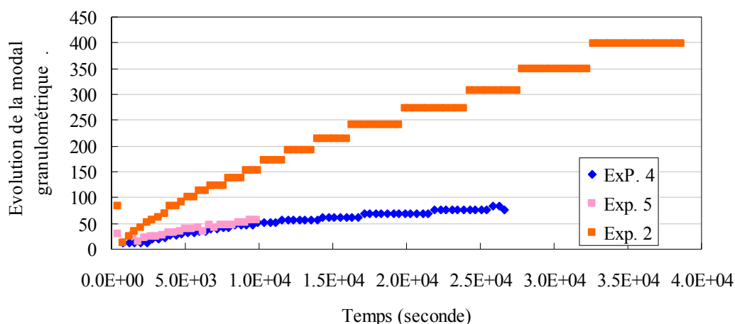
Figure V- 20: Influence de l'humidité relative sur l'évolution du mode granulométrique en fonction du temps
