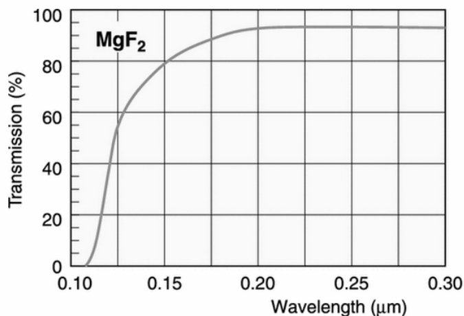
Figure III- 3 : Spectre de transmission de la fenêtre MgF 2
