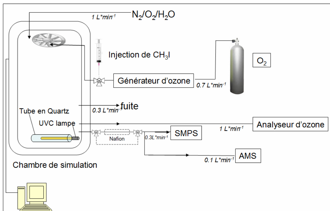
Figure V- 1 : Schéma du dispositif expérimental 13
