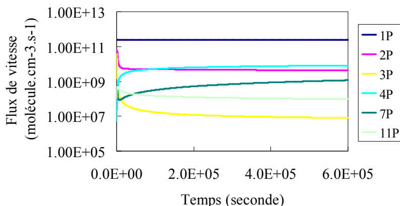
Figure IV- 2 : Flux de vitesse des réactions productrices de ·OH les plus importantes dans les conditions standards.
