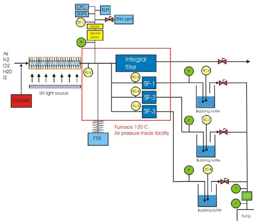
Figure II- 8 : schéma de l'installation expérimentale EXSI utilisée pour étudier la décomposition de I_2 et CH_3I sous UV et en présence de l'ozone
