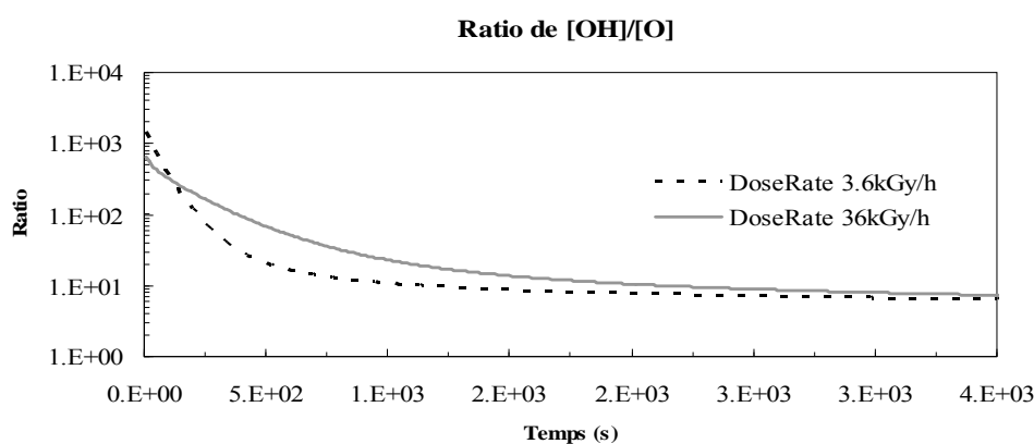
Figure II- 17 : Ratio de [\cdot\text{OH}] / [\cdot\text{O}] calculé avec le logiciel IODAIR (Température 90^\circ\text{C} , 80% HR, 1.7 bar, Débit de dose 3.6 et 36 kGy/h)
