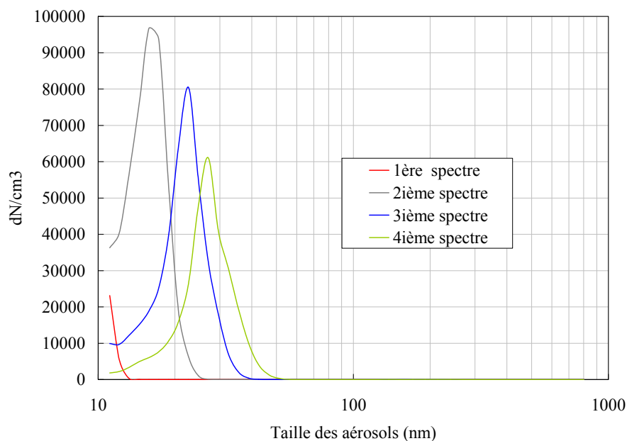
Figure V- 15 : Evolution de la distribution granulométrique de l'expérience 7 à partir du démarrage du générateur d'ozone
