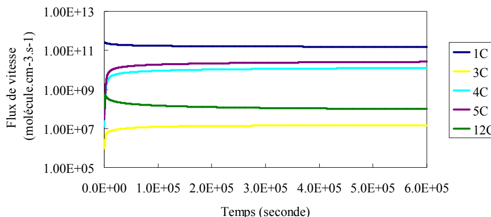
Figure IV- 3 : Flux de vitesse des réactions consommatrices de ·O, les plus importantes dans les conditions standards
