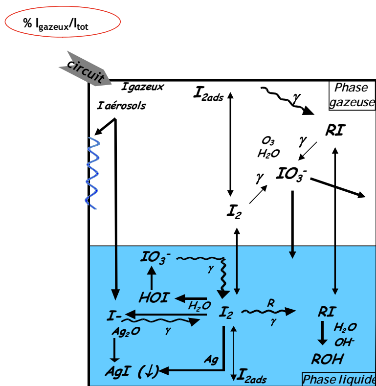
Figure II-5 : illustration de la compréhension actuelle de la chimie de l'iode dans une enceinte de confinement d'un réacteur en situation d'accident grave telle qu'intégrée dans le code ASTEC/IODE
