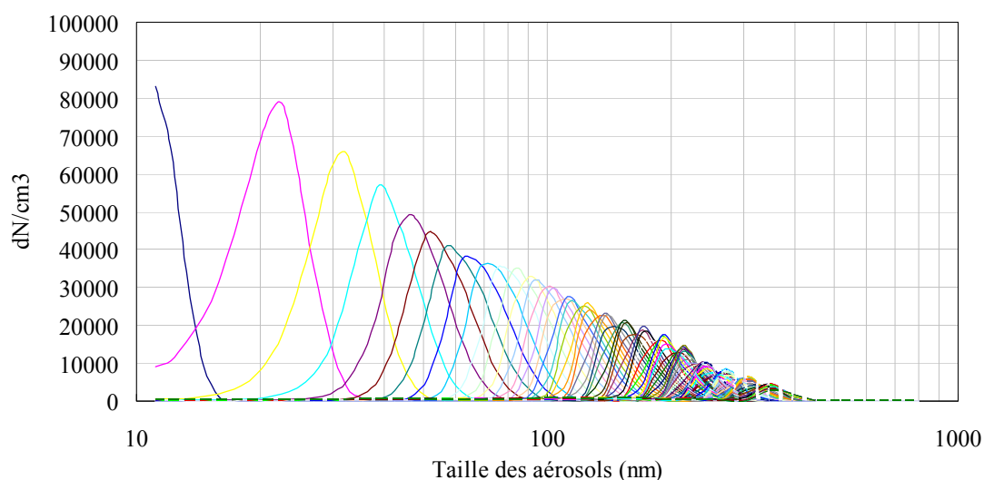
Figure V- 10 : Evolution de la distribution granulométrique des aérosol (en nombre, mesuré par le SMPS) pour l'expérience 2 ( \text{CH}_3\text{I} 15ppb, HR 60%, \text{O}_3 2ppm, à 30°C, avec photolyse) chaque courbe représente un scanne de SMPS (de 6 min 42 s).
