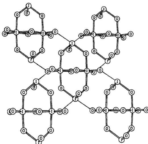
Figure V- 31 : Structure de I_4O_{12} avec deux contacts intermoléculaires entre chaque maille
