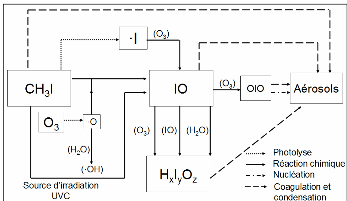
Figure V- 13 : Schéma réactionnel simplifié de la formation des aérosols d'oxydes d'iode dans la chambre de simulation, dans nos conditions expérimentales
