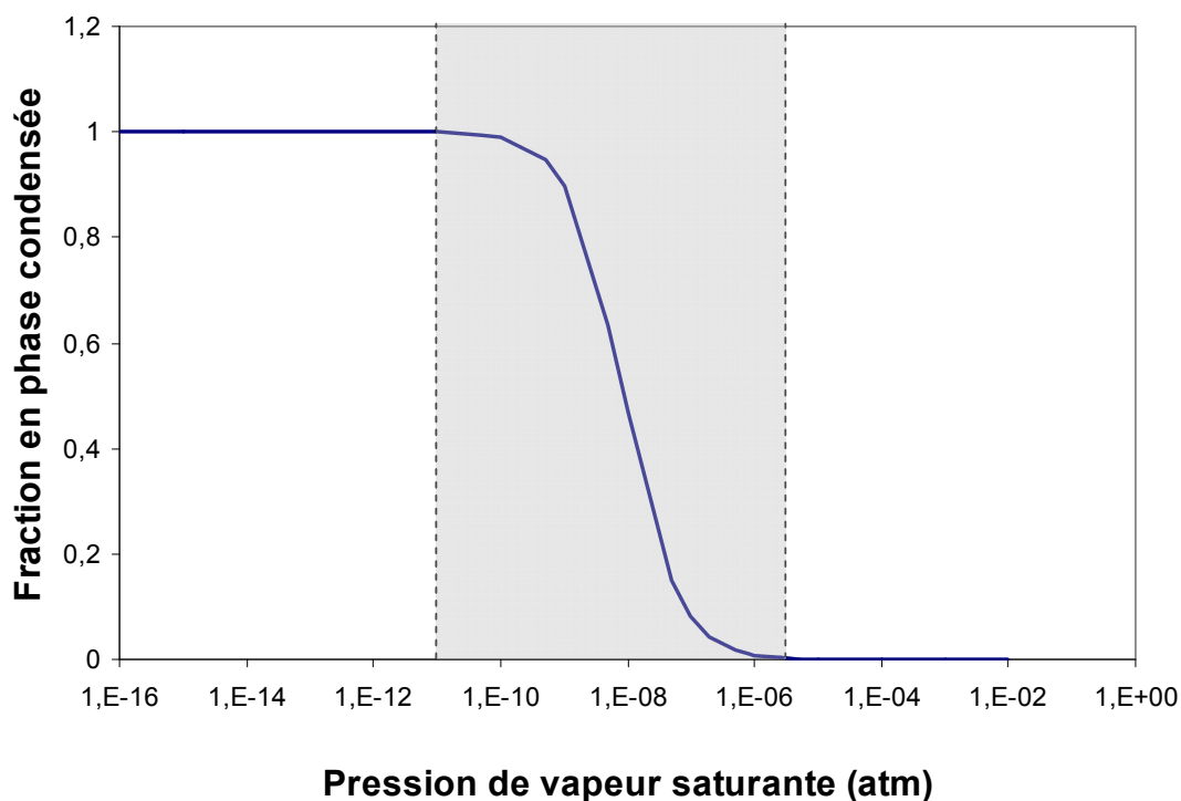
Figure V- 36 : Fraction \xi_{\text{aer},i} d'une espèce i semi-volatile en phase condensée à l'équilibre thermodynamique avec la phase gazeuse, en fonction de sa pression de vapeur saturante dans les conditions de l'expérience 9, à t_{\text{max}} ( T = 30^\circ\text{C} , C_{\text{aer}} = 69.23 \mu\text{g}/\text{m}^3 , et en supposant M_{\text{aer}} = 200 \text{ g/mol} ).
