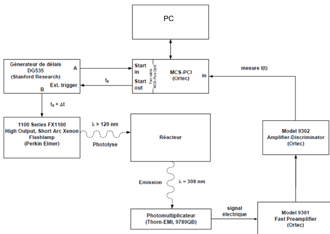
Figure III- 6 : Schémas du système de détection et de contrôle
