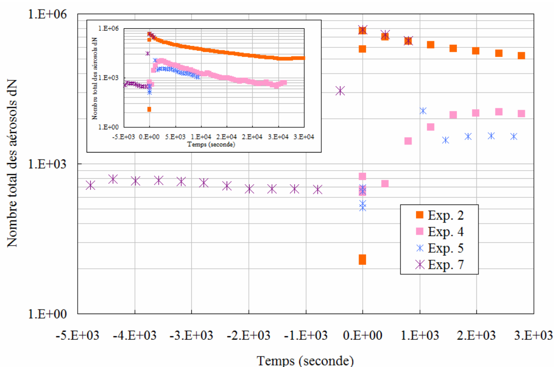
Figure V- 19: Influence de l'humidité relative sur la cinétique d'apparition des particules pour les expériences 2, 7 (HR 60%) et 4, 5 (HR 15%). L'évolution de nombre total des aérosols durant le temps total en haut à gauche.
