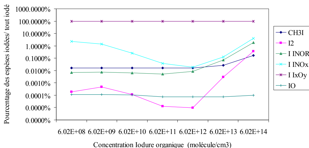
Figure IV- 9 : Pourcentages moyens des espèces iodées sur le temps total en fonction de la concentration initiale des iodures organiques à plus longue chaîne, à 90°C, humidité relative à 80% et débit de dose de 3.6kGy/h
