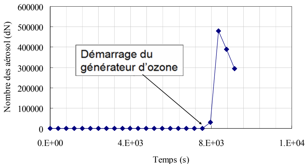
Figure V- 16 : Evolution du nombre total d'aérosols lors de l'expérience 7
