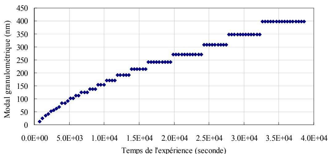
Figure V- 11 : Evolution en fonction du temps de la distribution granulométrique modale pour l'expérience 2
