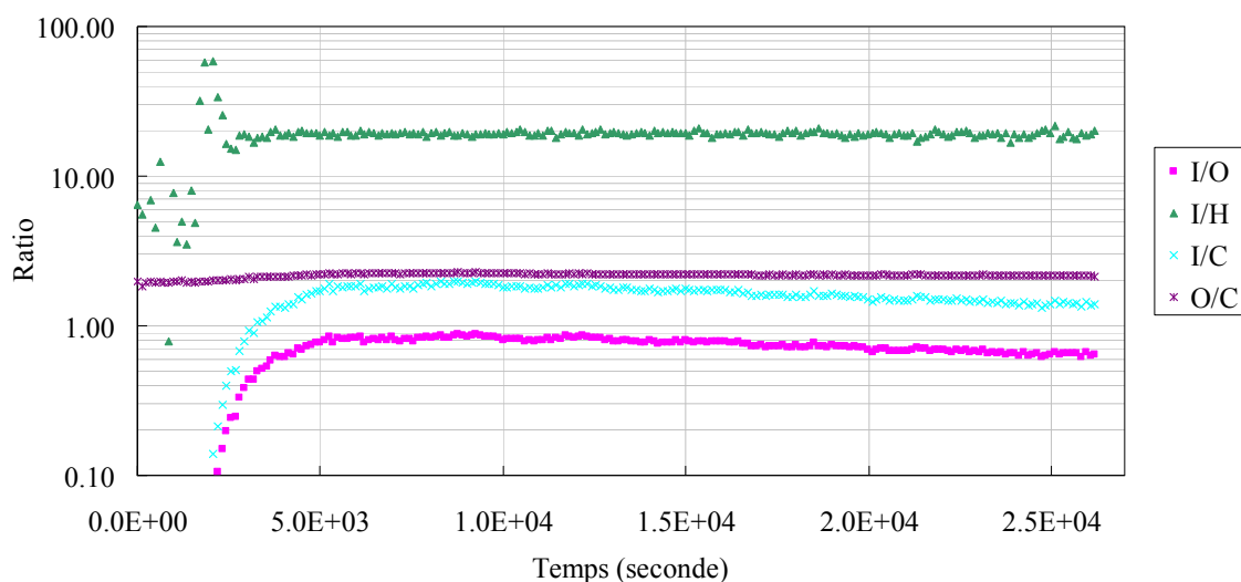
Figure V- 29 : Rapport des éléments constituant les aérosols en fonction du temps lors de l'expérience 9
