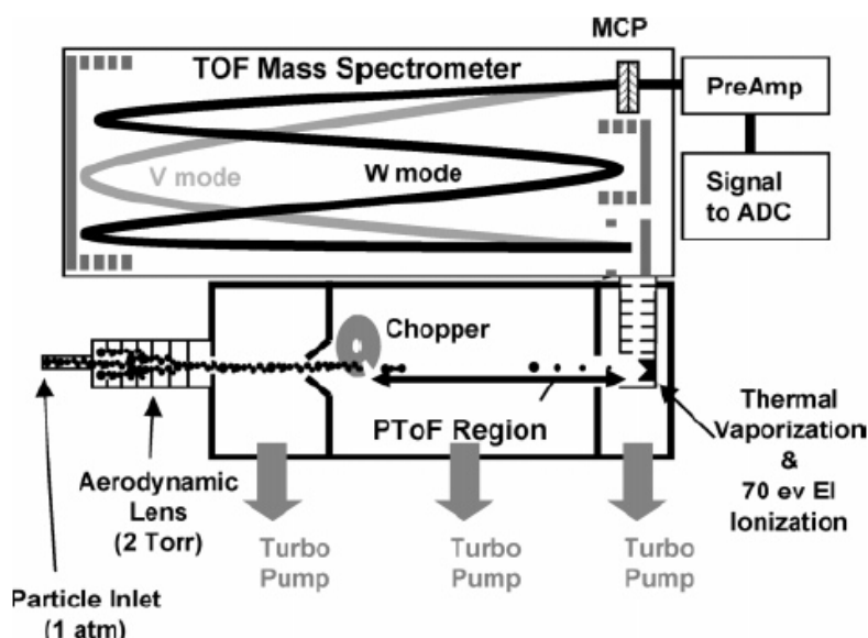
Figure V- 7 : Schéma de principe du HR-ToF-AMS (DeCarlo, Kimmel et al. 2006)
