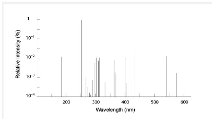
Figure V- 2: Spectre 14 de la lampe à vapeur de mercure basse pression
