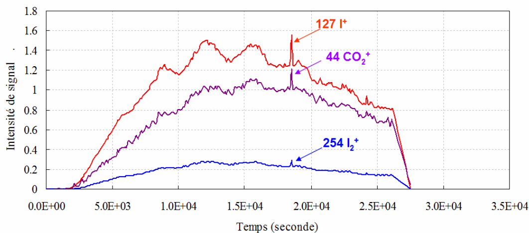
Figure V- 25 : Evolution des fragments les plus intenses ( I^+ , CO_2^+ et I_2^+ ) en fonction du temps lors de l'expérience 9
