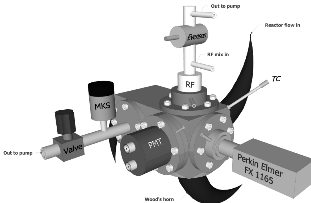
Figure III- 5 : les positions de la lampe flash, de la lampe fluorescente et du PMT
