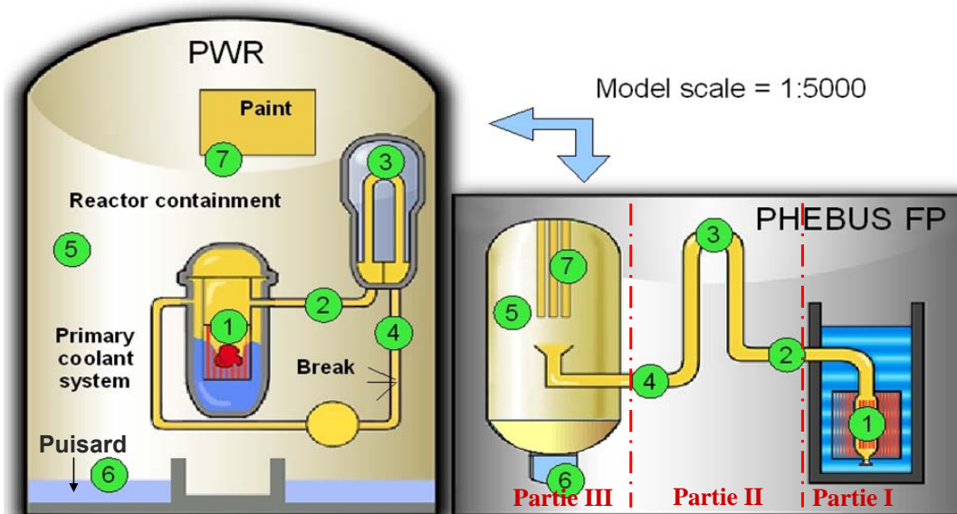
Figure II- 1 : Illustration d'un REP (gauche) et de l'installation PHEBUS-PF (droite)
