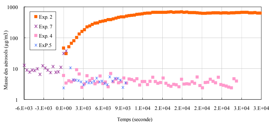
Figure V- 18: Influence de l'humidité relative sur la concentration massique des aérosols (en considérant une densité de 4 \text{ g/cm}^3 , d'après Jimenez et al., 2003) pour les expériences 2, 7 (HR 60%) et 4, 5 (HR 15%)
