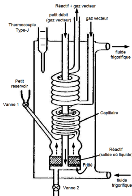
Figure III- 2 : le système d'injection (haut) comprenant deux saturateurs (bas)
