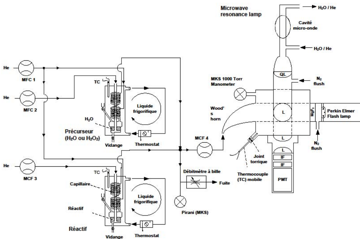
Figure III- 1 : Système Flash Photolyse – Résonance Fluorescente
