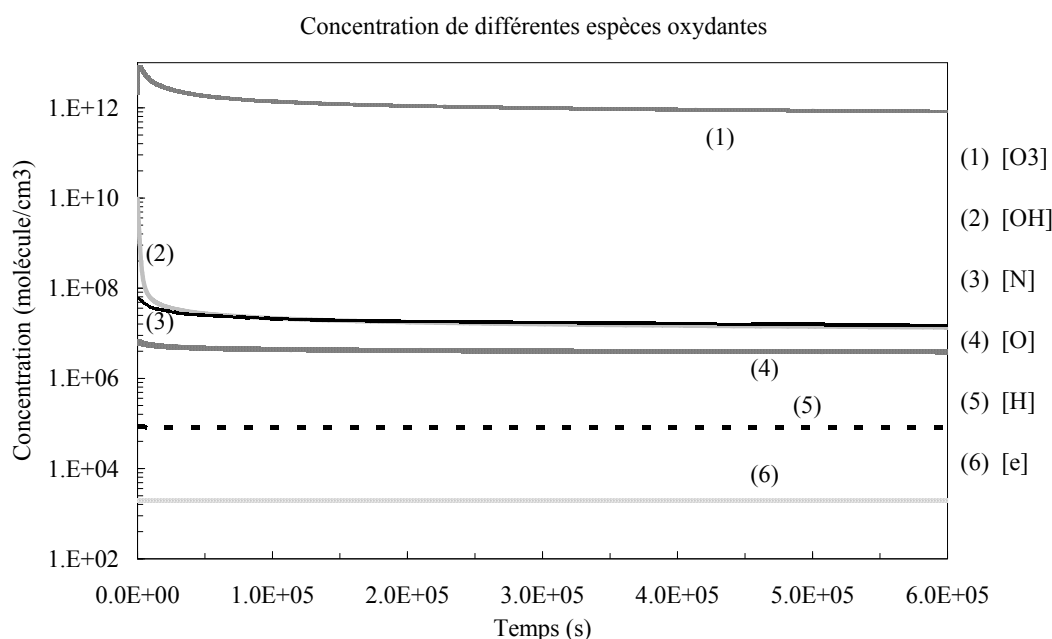
Figure II- 18 : Evolution de différents produits radiolyse de l'air dans l'enceinte de confinement accidenté (Température 90°C, 80% HR, 1.7 bar, Débit de dose 3.6kGy/h)
