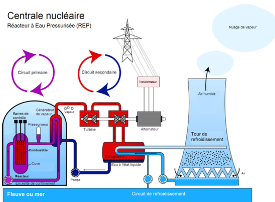
Figure I- 1 Schéma de principe d'une tranche nucléaire disposant d'un REP 3
