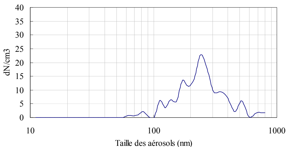
Figure V- 9 : Distribution granulométrique en nombre d'un blanc dans la chambre (mesurée par le SMPS), réalisé avant l'expérience 2
