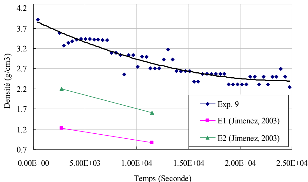
Figure V- 33 : Densité des aérosols d'oxydes d'iode en fonction du temps
