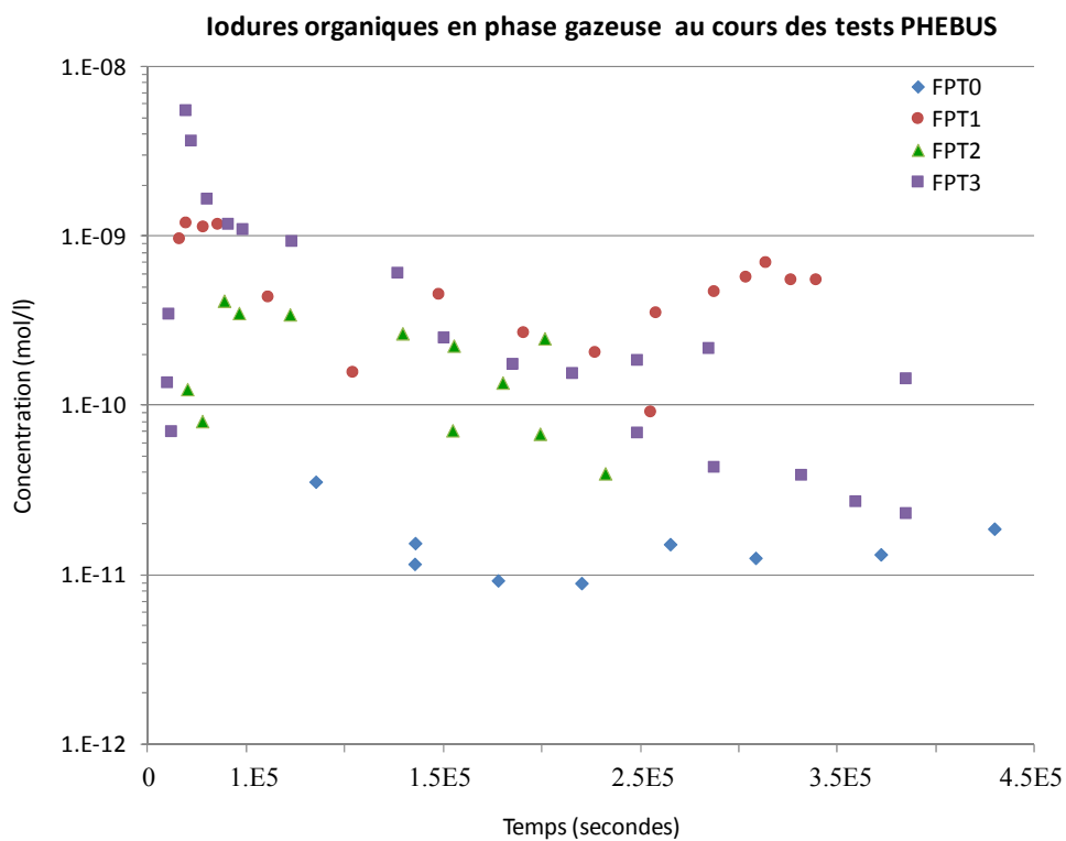
Figure II-3 : concentration d'iodures organiques dans l'enceinte PHEBUS pour FPT0, FPT1, FPT2 et FPT3 ( 1.10^{-8} \text{mol.L}^{-1} = 0.224 \text{ppm} à 1 atm)
