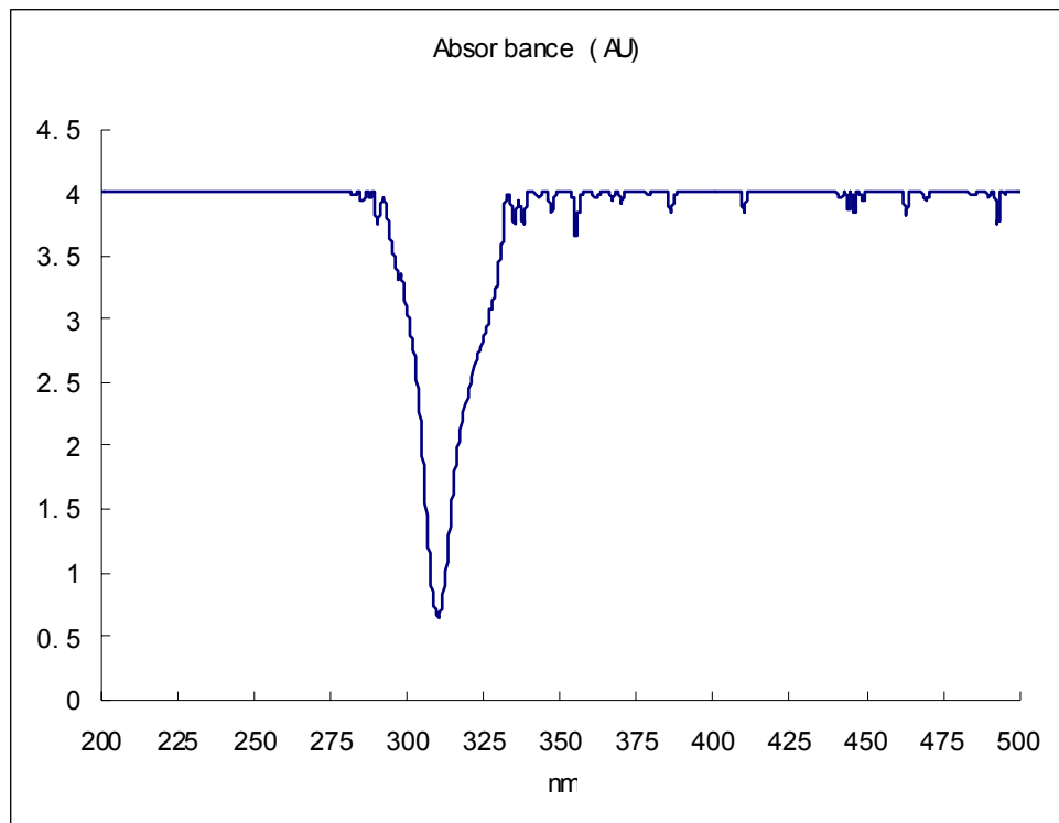
Figure III- 7 Spectre d'absorption du filtre
