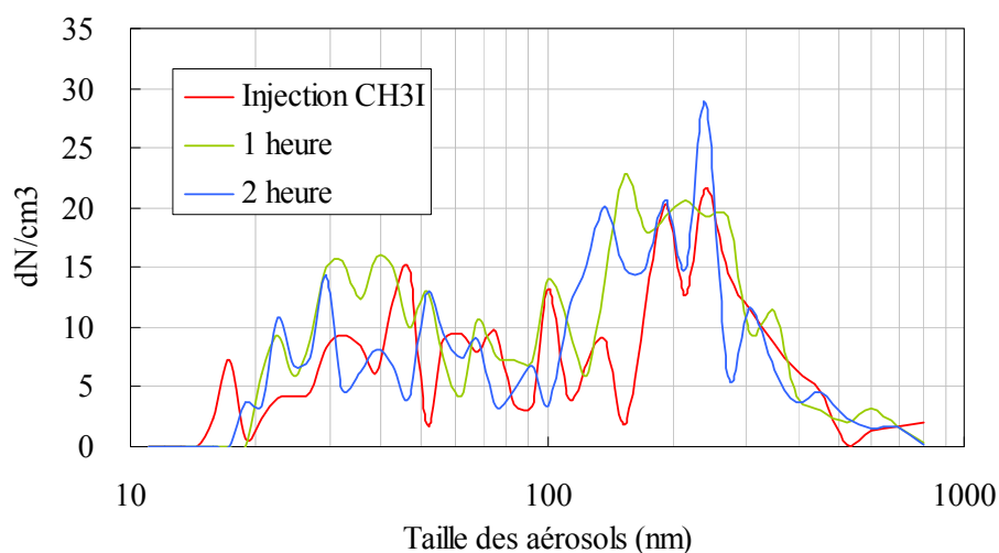
Figure V-14 : Evolution de la distribution granulométrique de l'expérience 7 lorsque la concentration résiduelle d'ozone est de 0.07ppm (générateur d'ozone éteint)
