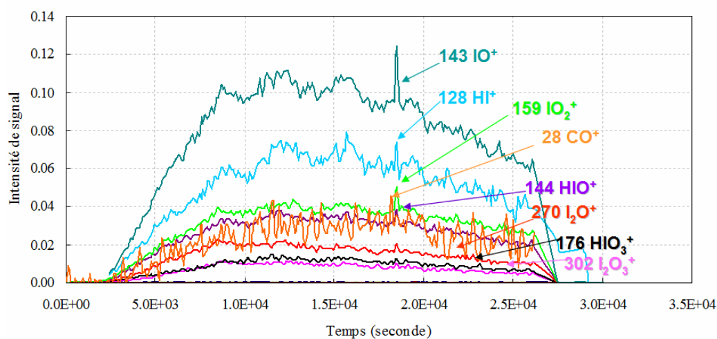
Figure V- 26 : Evolution des fragments IO^+ , CO^+ , HI^+ , IO_2^+ , HIO^+ , I_2O^+ , HIO_3^+ et I_2O_3^+ en fonction du temps lors de l'expérience 9
